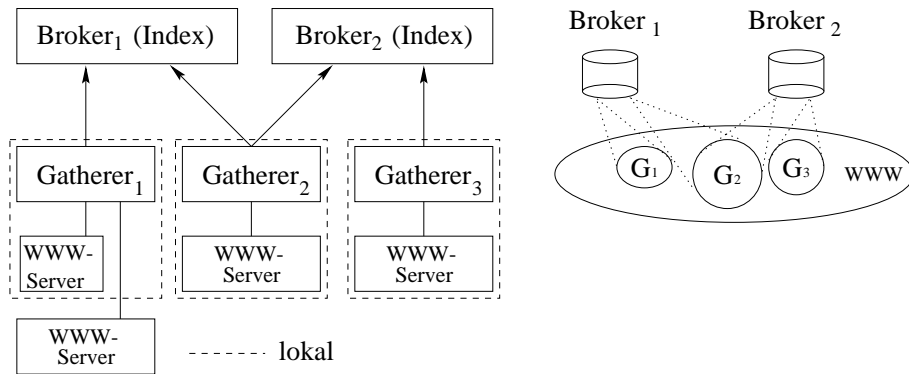
Abbildung 4.2: Gemeinsame Nutzung eines Gatherers
