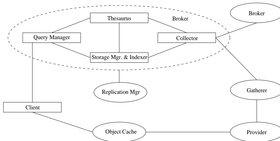
Abbildung 3.1: Harvest Architektur [HSW96]
