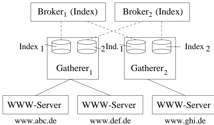
Abbildung 4.4: Zusammenfassung der Indizes nach DDC: Die Gatherer erzeugen je Thematik einen Index (Index 1 und Index 2 ), der vom Broker, der die zu einer Thematik gehörenden Dokumente indiziert, gelesen wird.
