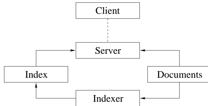
Abbildung 3.6: freeWAIS Architektur
