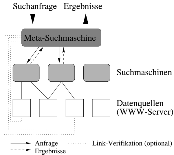
Abbildung 1.3: Meta-Suchmaschine
