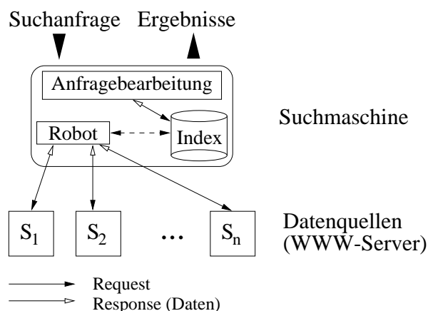
Abbildung 1.2: einfache Suchmaschine
